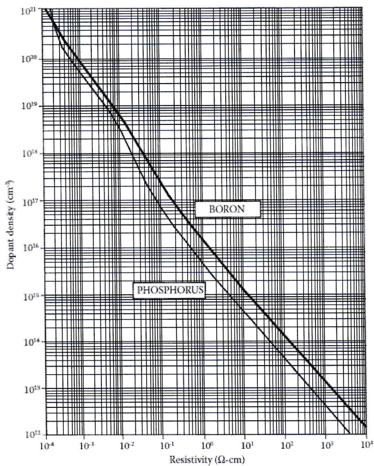
Figure : (Log-Log) Résistivité en \Omega\cdot\text{cm} en fonction de la concentration d'impuretés/cm 3 dans le silicium
