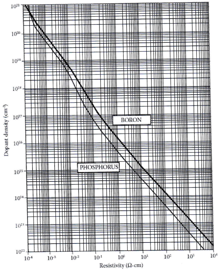
Figure : (Log-Log) Résistivité en \Omega\cdot\text{cm} en fonction de la concentration d'impuretés/ \text{cm}^3 dans le silicium
