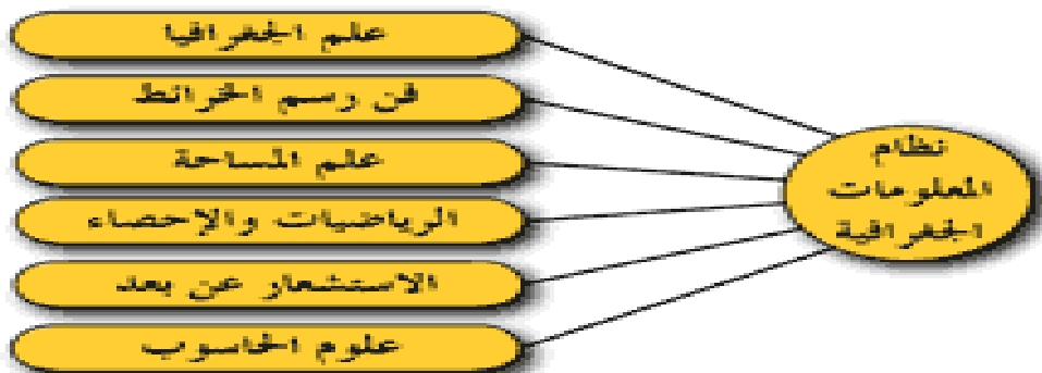
شكل رقم 01: علاقة نظم المعلومات الجغرافية بالعلوم الأخرى
